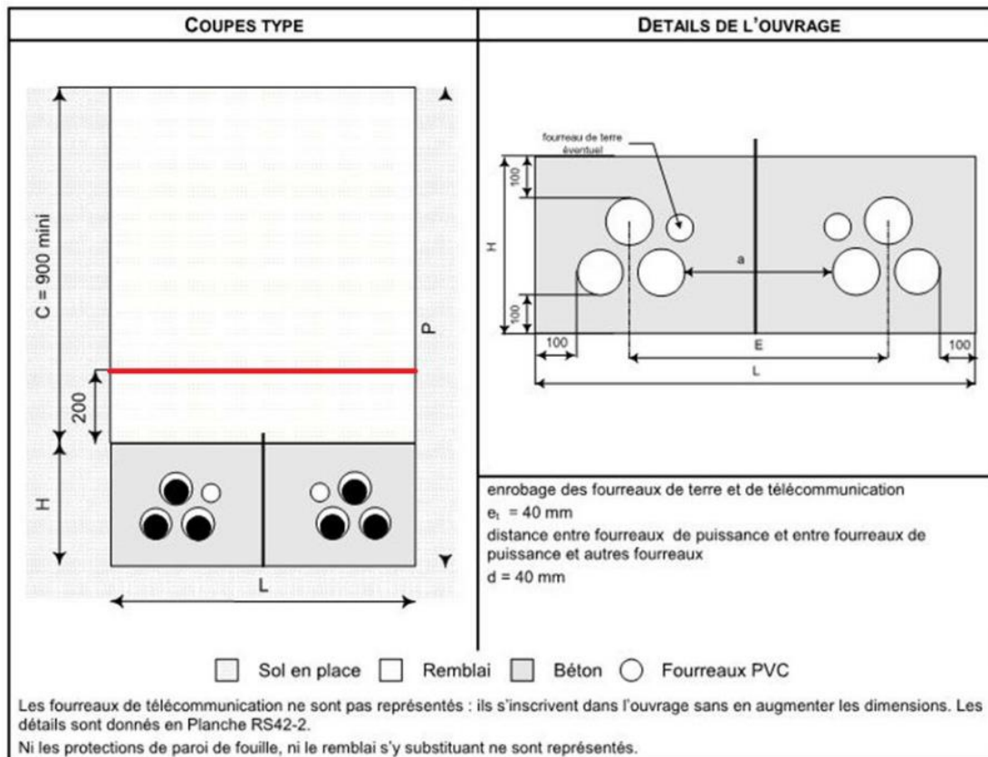
Figure 11: Mode de pose de fourreaux en double trèfle
