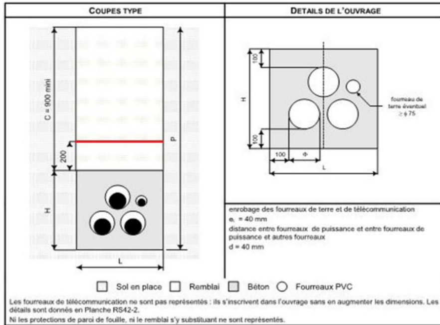
Figure 10: Mode de pose de fourreaux en simple trèfle
