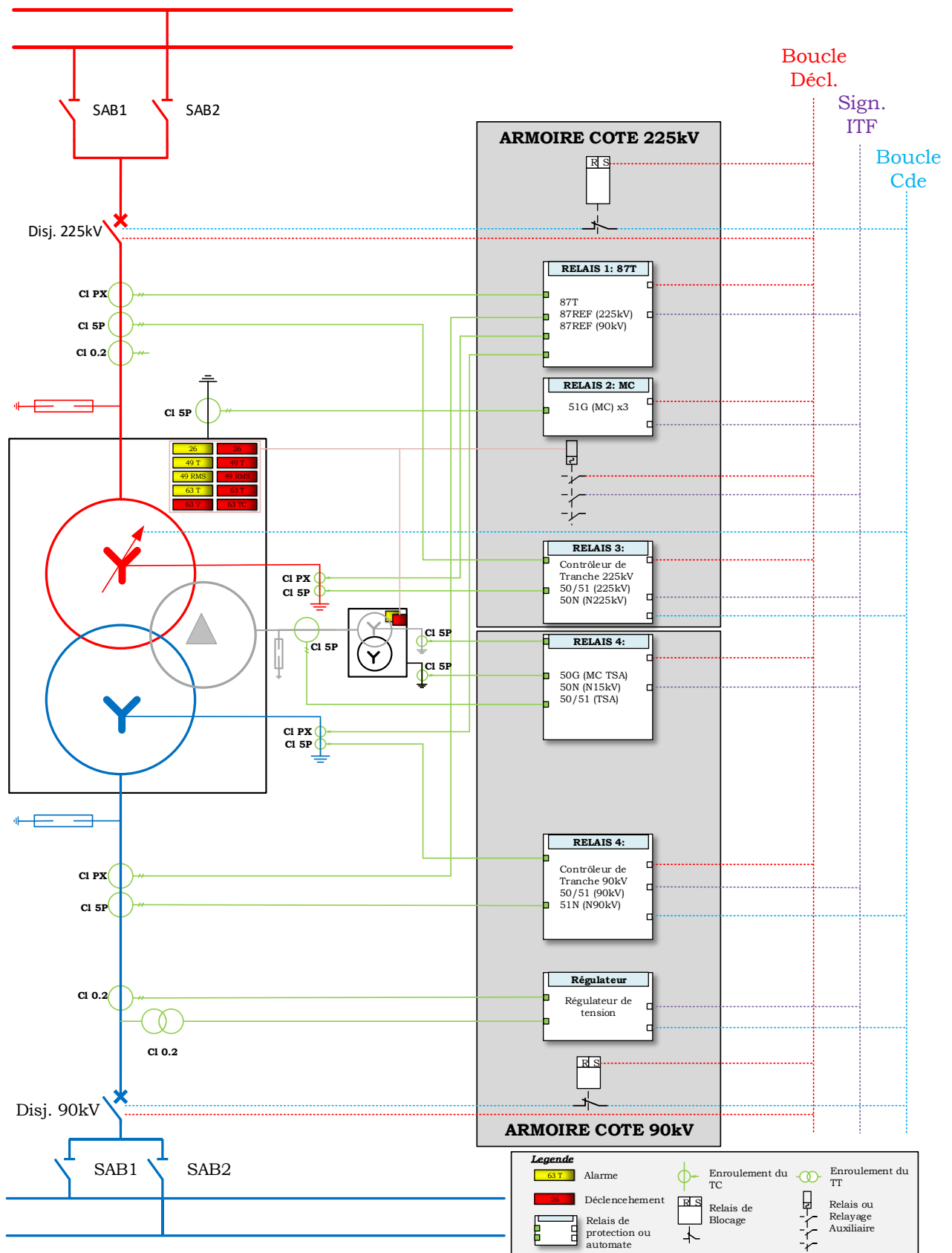
Figure 4 : Schéma logique plan de protection transformateur HT/HT
