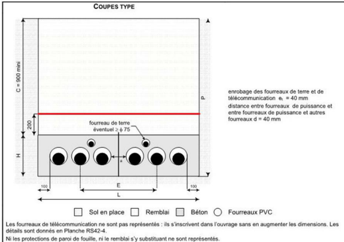
Figure 13 : Mode de pose de fourreaux en double nappe
