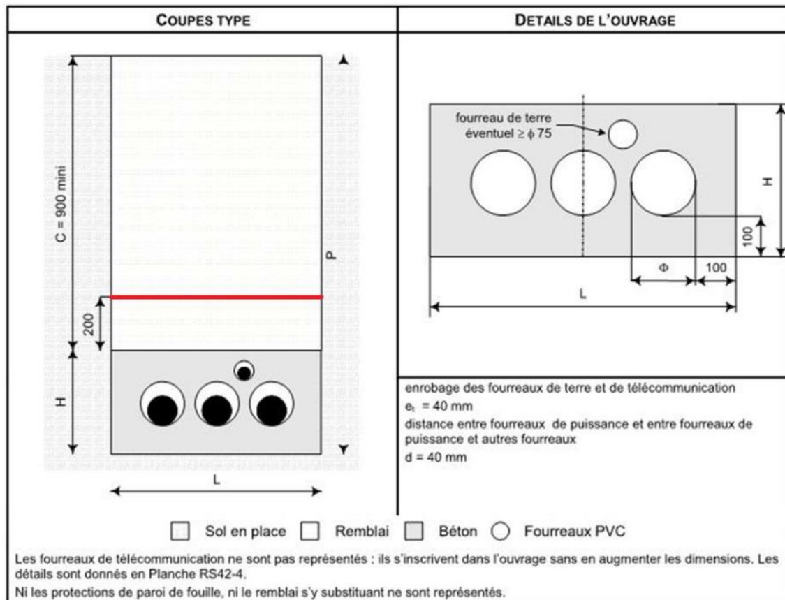
Figure 12: Mode de pose de fourreaux en nappe
