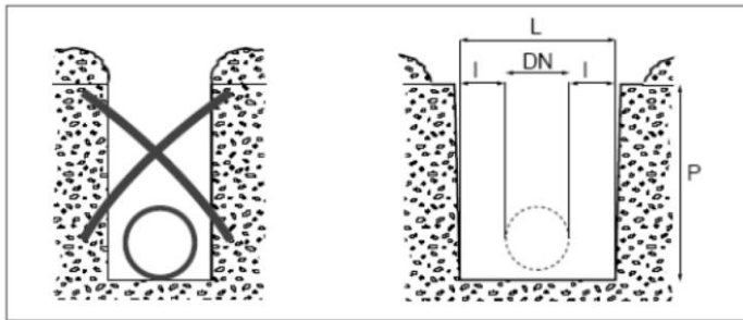
Figure 6 : Largeur minimale des tranchées
