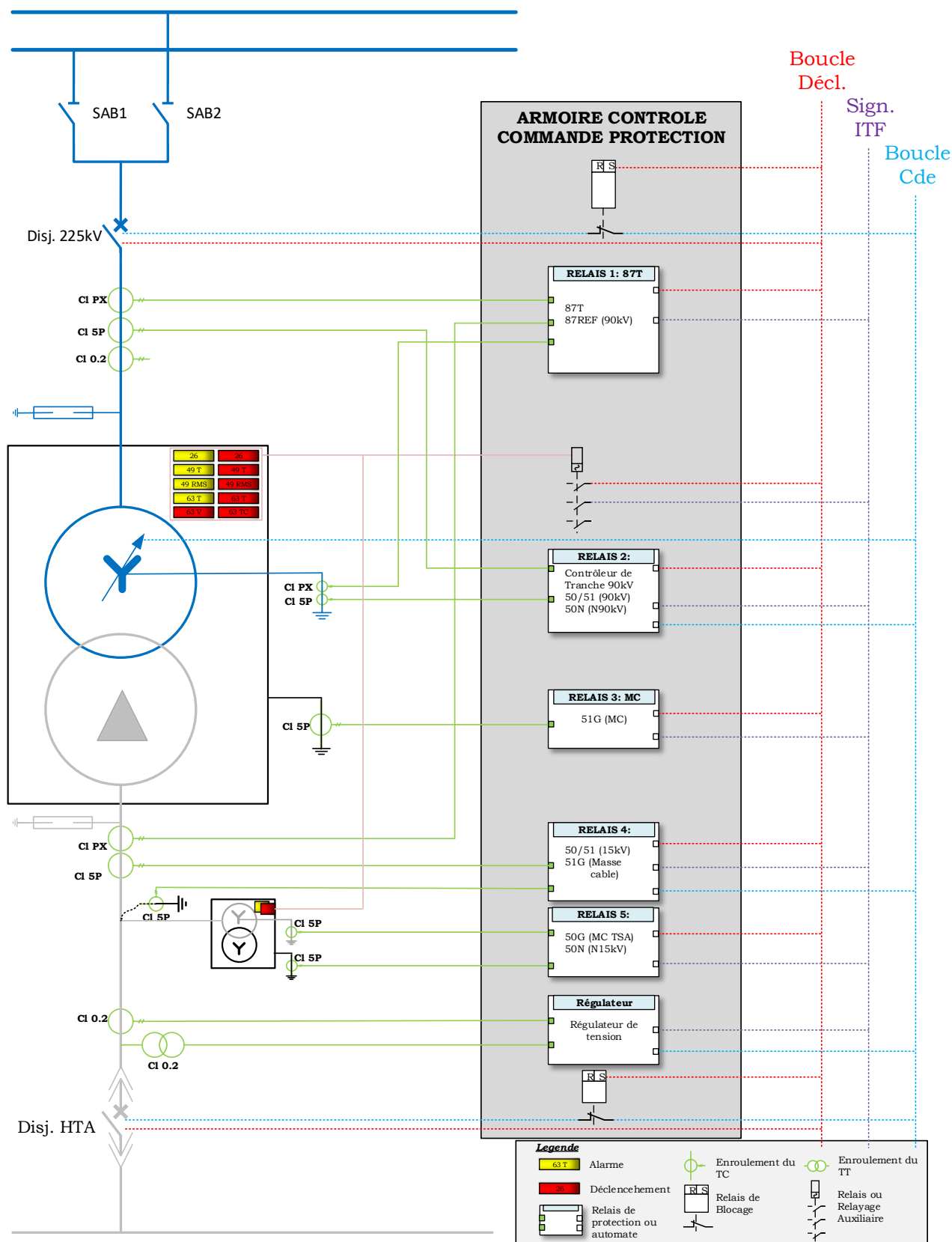
Figure 5 : Schéma logique plan de protection transformateur HT/MT
